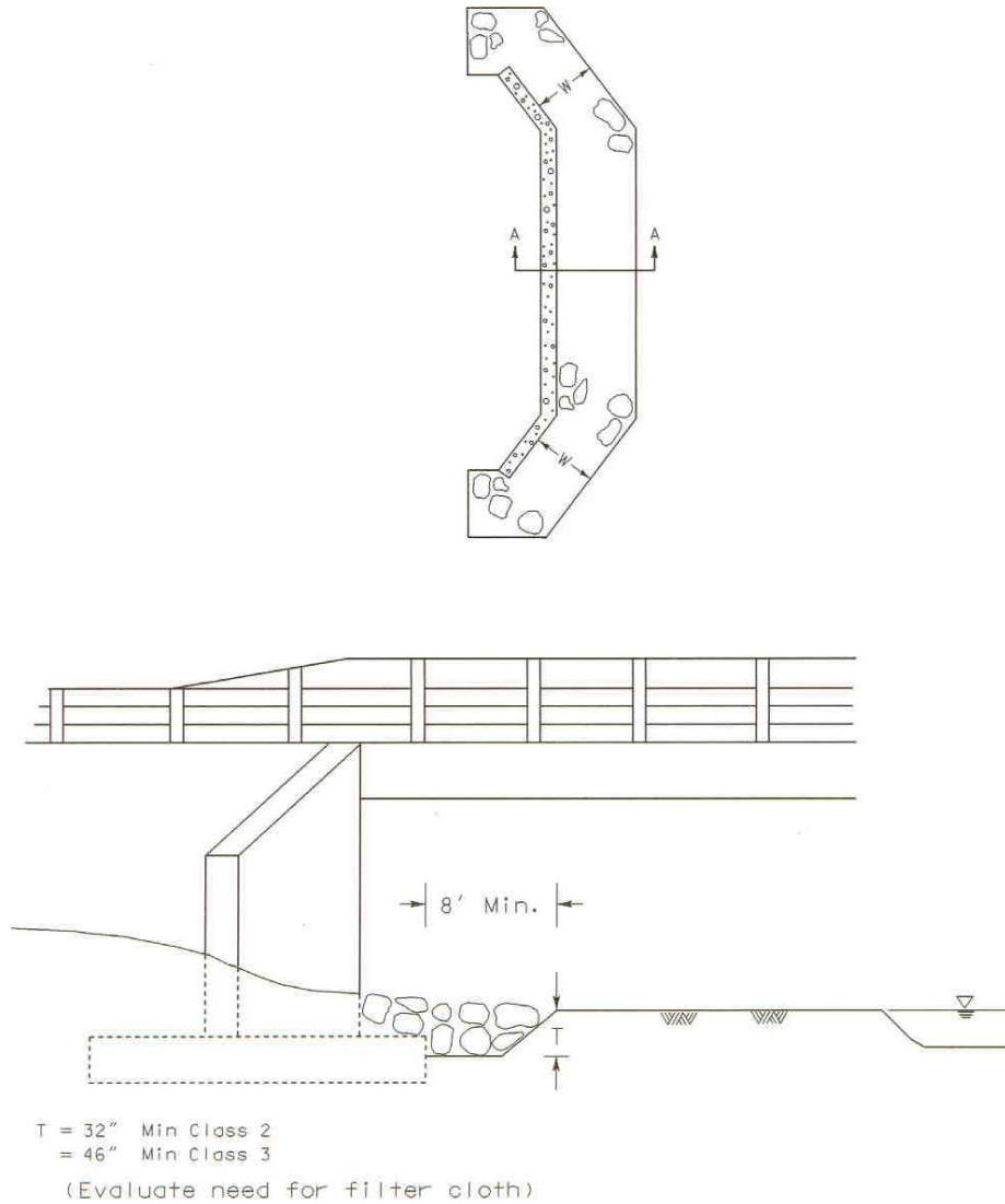
Section A-A
